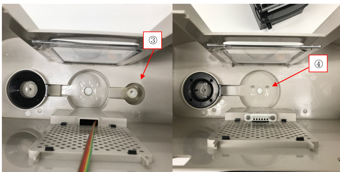
液面検知センサーの変更（③フロートスイッチ式 ⇒ ④電極センサー式）
